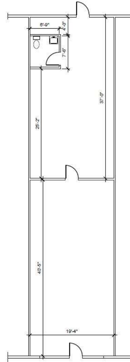
2029 - FLOOR PLAN SCALE: 1/8" = 1'-0"
