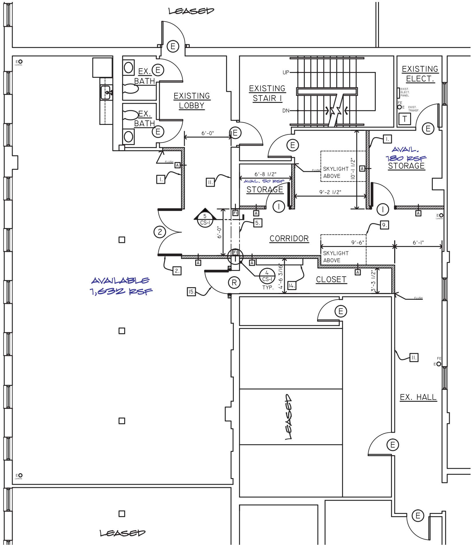
1 PARTIAL FLOOR PLAN 3. 4. 6. 7. 8. 10. 12. A-2 1/4"=1'-0"
