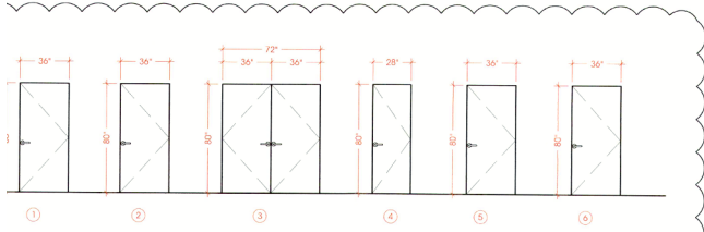
DOOR SCHEDULE
