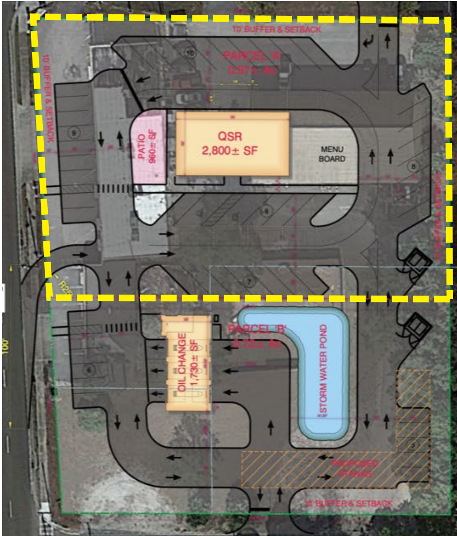
QSR LAYOUT
