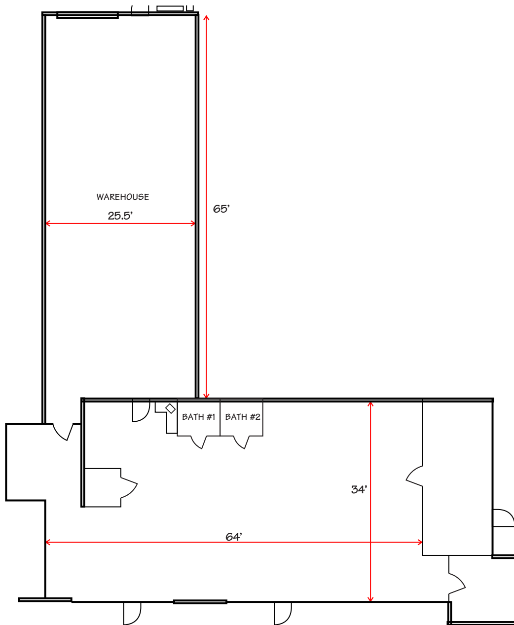
SUITE 108 4,342 SF
