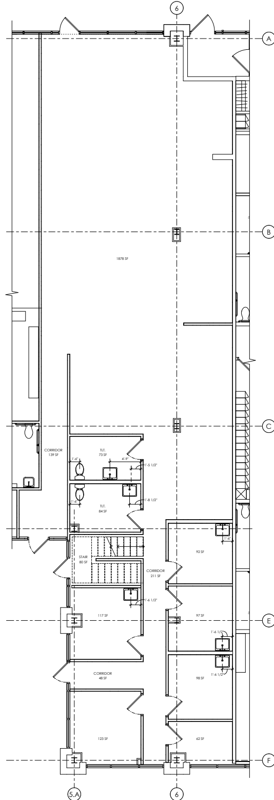
1 TENANT E - FIRST FLOOR
