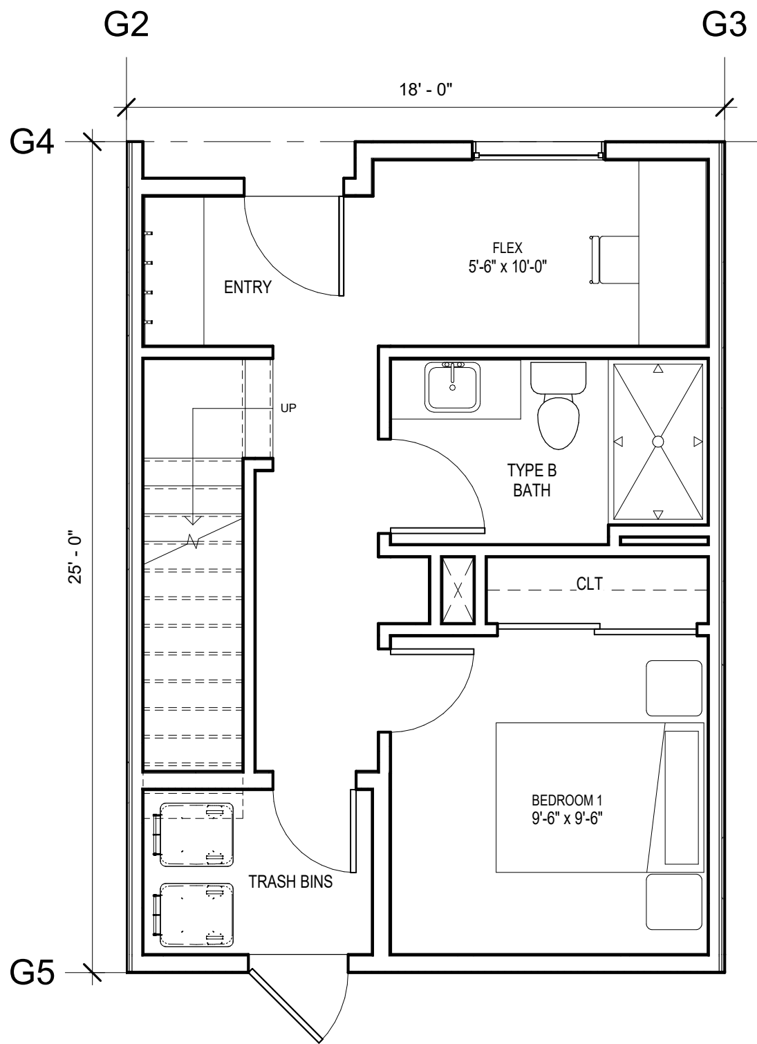
1 UNIT TYP L1 1/4" = 1'-0"
