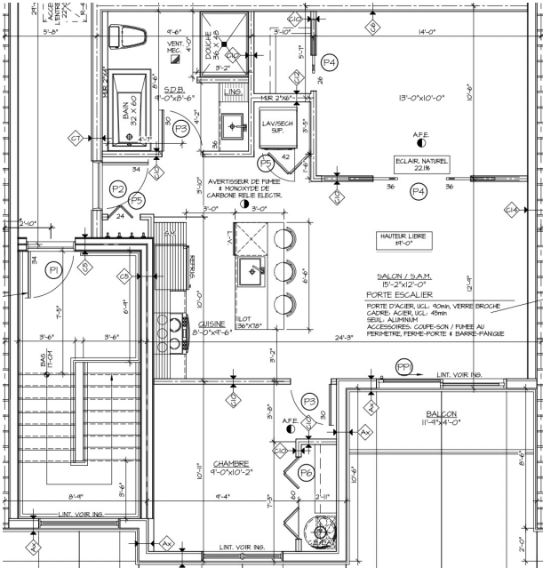
191-A Ch Old Chelsea - Unit 105/Unité 105
