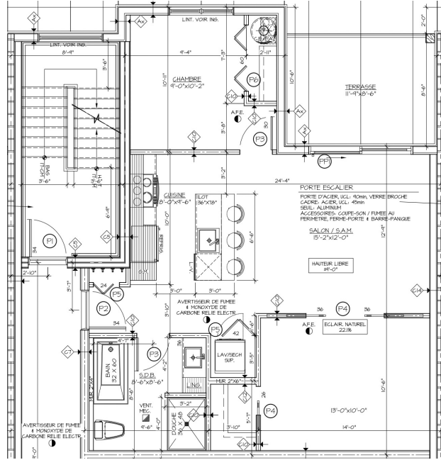
191-A Ch Old Chelsea - Unit 104/Unité 104
