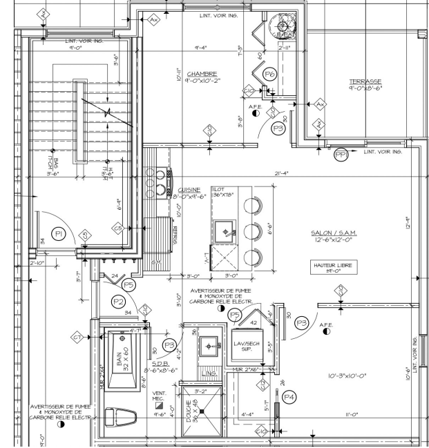
191-B Ch Old Chelsea - Unit 104/Unité 104
