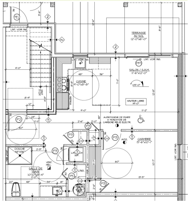
189 Ch Old Chelsea – Unit 102/Unité 102
