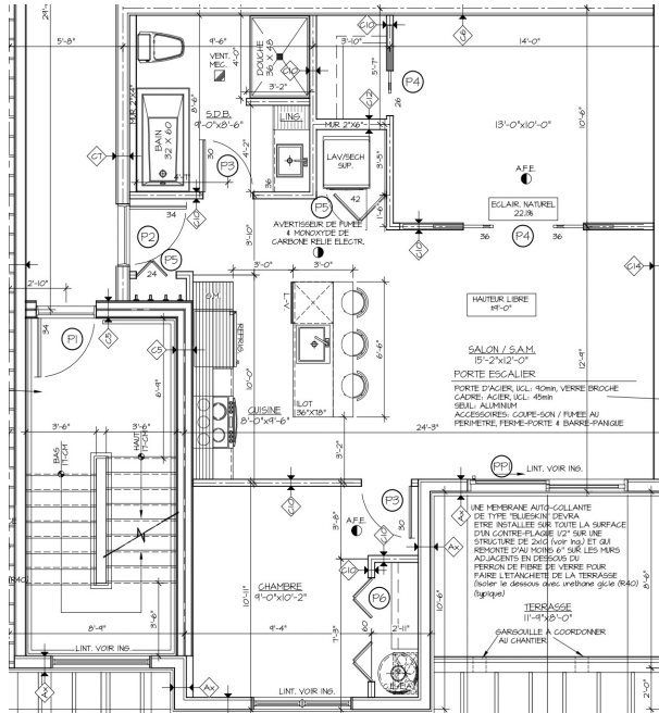
191-A Ch Old Chelsea - Unit 103/Unité 103
