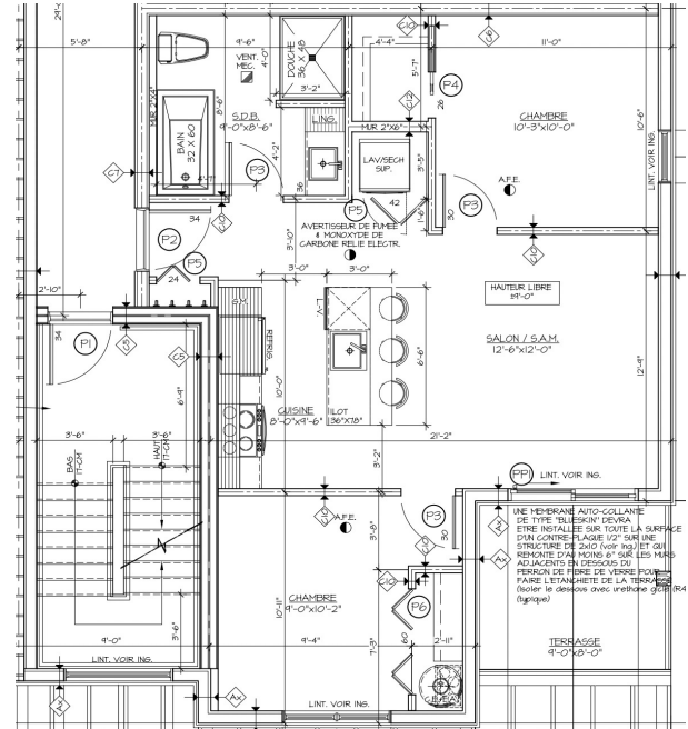
191-B Ch Old Chelsea - Unit 103/Unité 103
