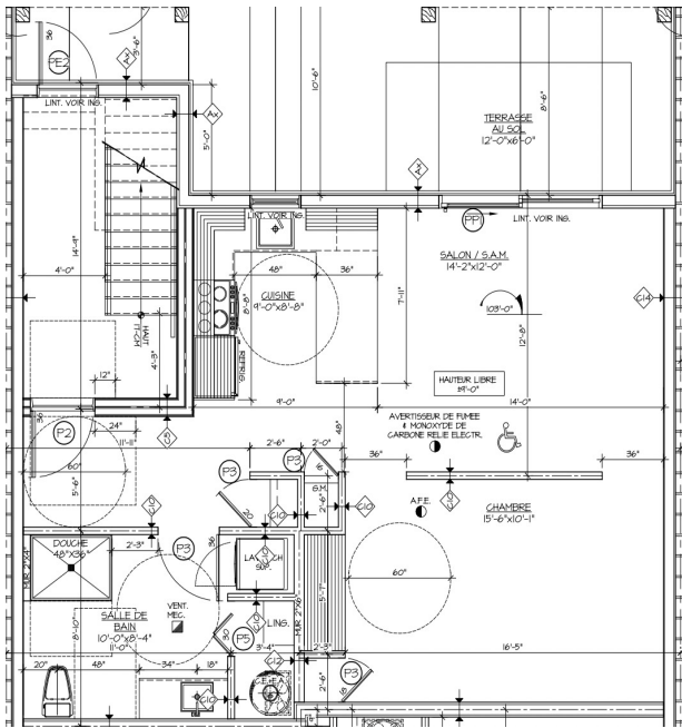
191-A Ch Old Chelsea – Unit 102/Unité 102
