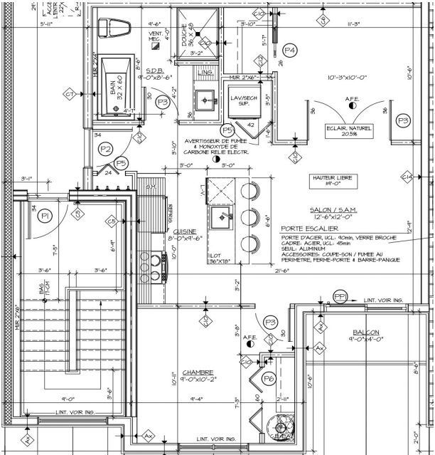
189 Ch Old Chelsea - Unit 105/Unité 105
