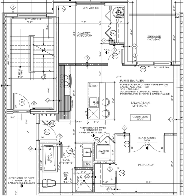
189 Ch Old Chelsea - Unit 104/Unité 104
