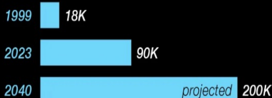
DTLA Population
