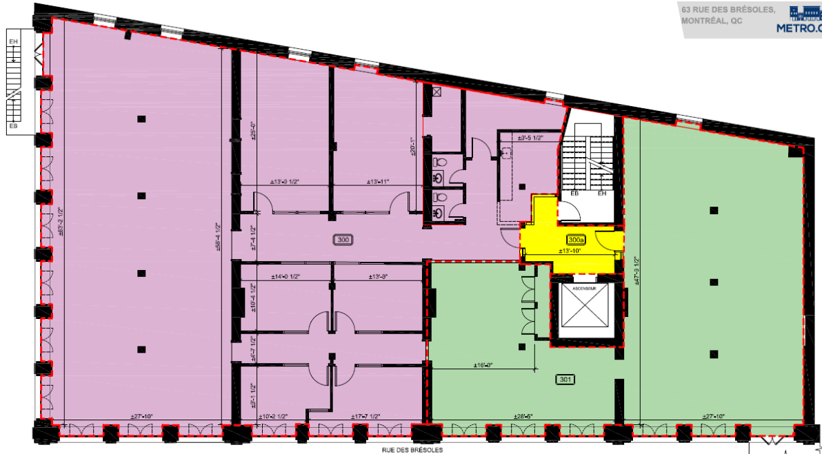
PLAN DE LOCATION- 4e ÉTAGE SCALE / ÉCHELLE: 1/8" = 1'-0"
