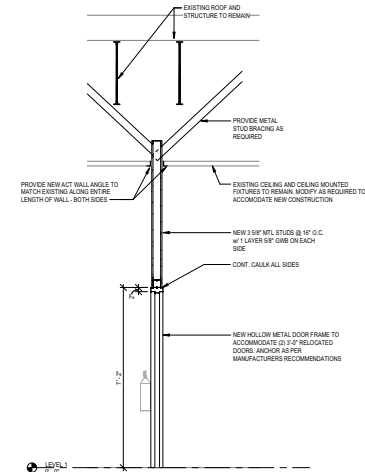
4 WALL SECTION SCALE: 1/2" = 1'-0"
