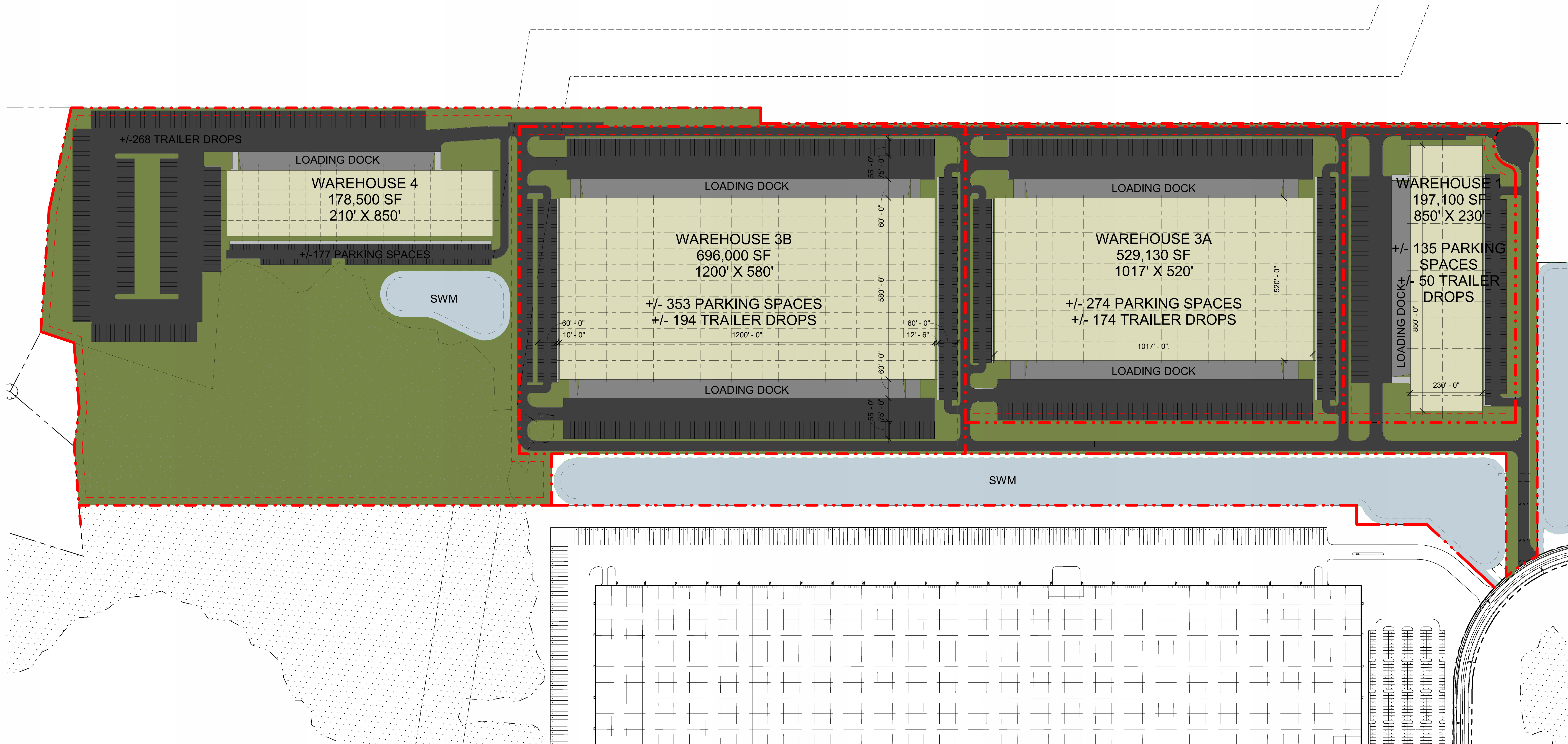
1 SITE PLAN - OPTION 13C 1 : 1600
