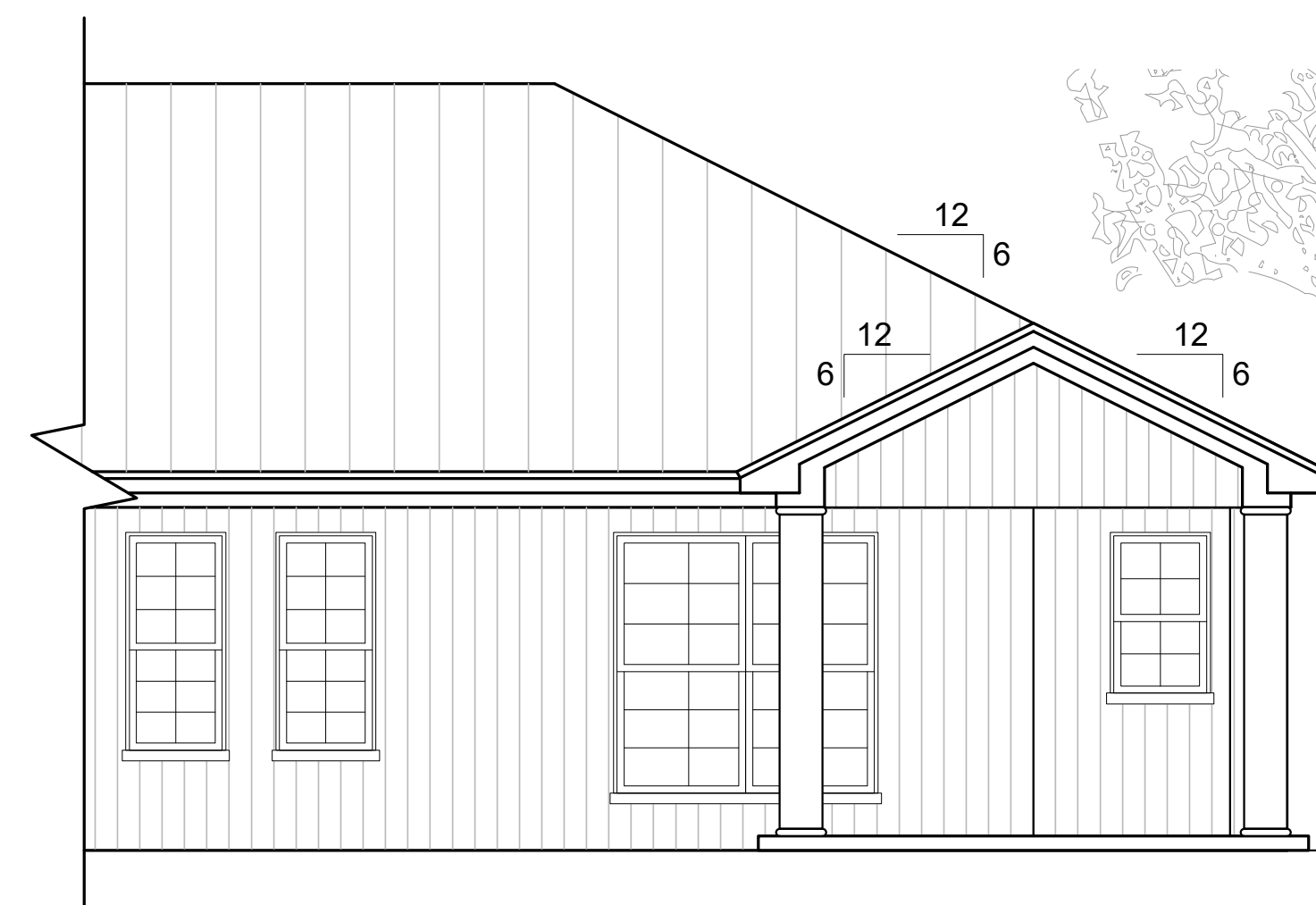
4 ELEVATION 490-11, 490-12, 161-11, 161-12, 166-5 & 166-6
