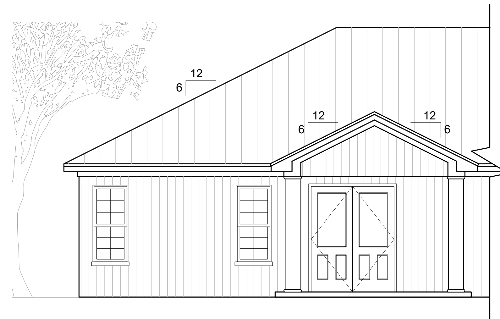
2 ELEVATION 490-1, 490-22, 161-1, 161-22, 436-1 & 436-12
