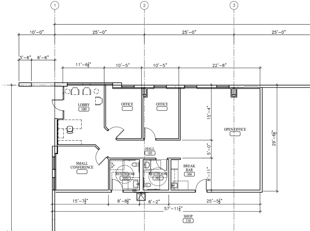
01 OFFICE PLAN SCALE: 1/8" = 1'-0"
