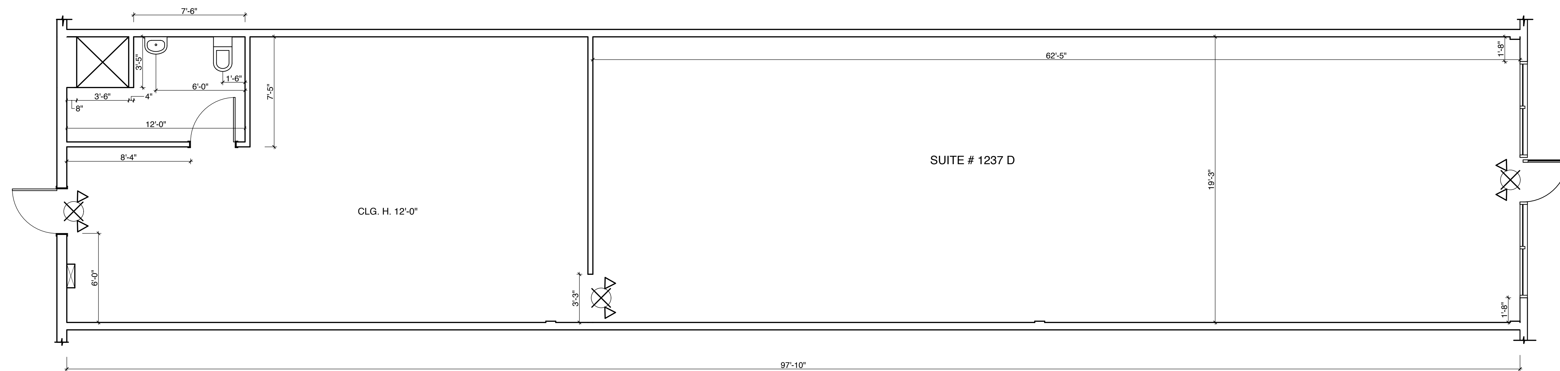
1 A-1 FLOOR PLAN SCALE: 1/4" = 1'-0"
