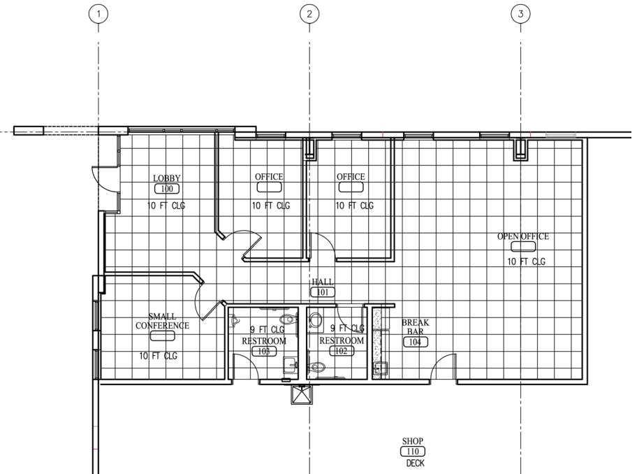
02 RCP SCALE: 1/8" = 1'-0"
