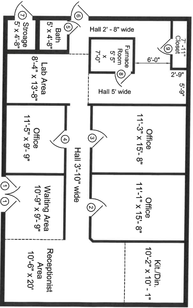
Floor Plan Scale: 1/8" = 1'
