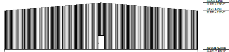
4 RIGHT ELEVATION A2 SCALE: 1/8" = 1'-0"
