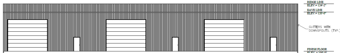
2 REAR ELEVATION A2 SCALE: 1/8" = 1'-0"
