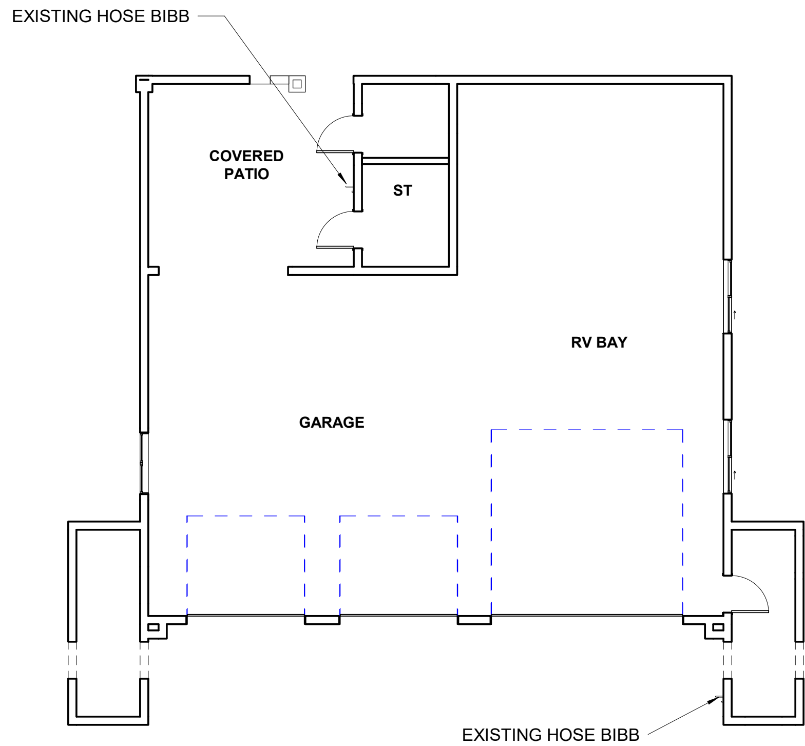
3 EXISTING GARAGE SCALE: 1/8" = 1'-0"
