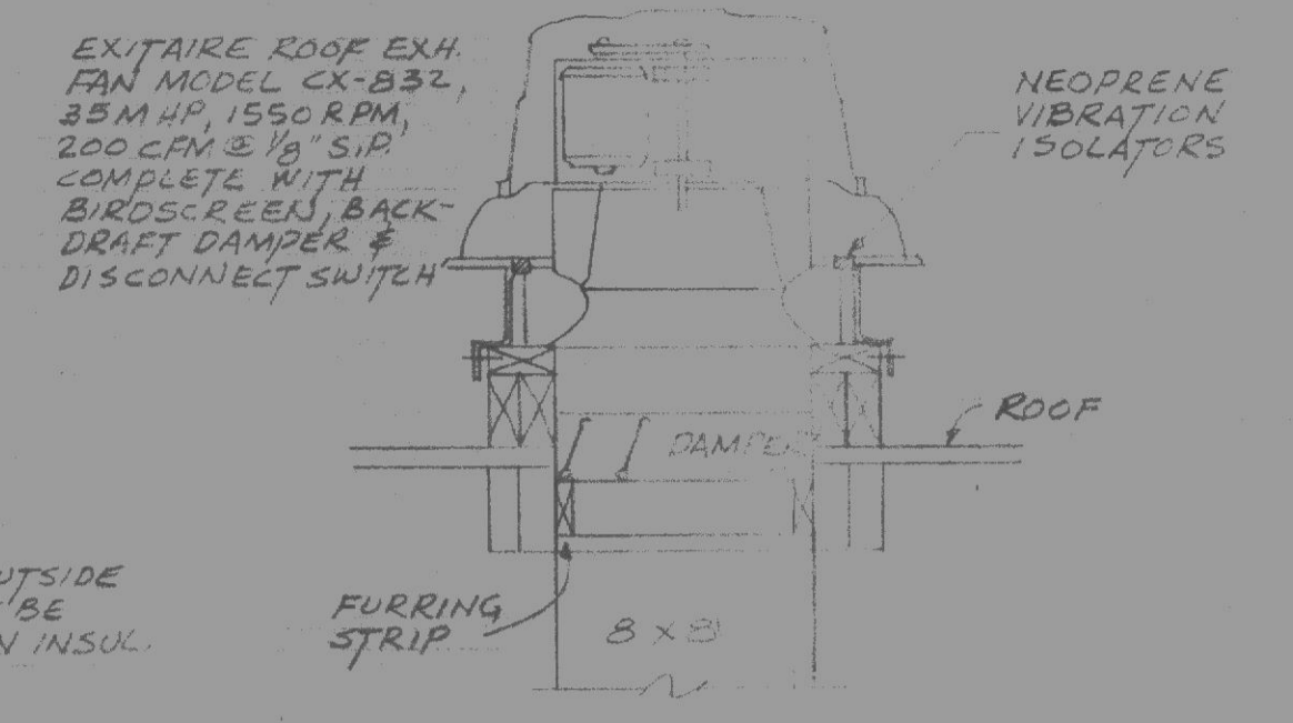
TOILET ROOM EXH. FAN DETAIL NO SCALE
