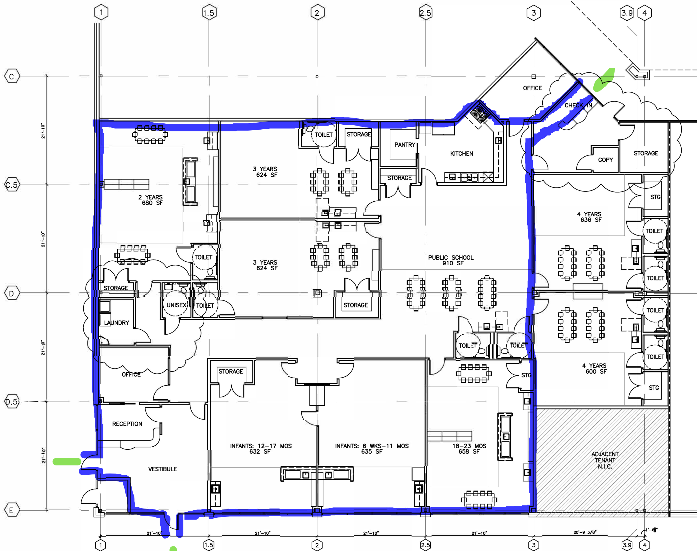
FLOOR PLAN SCALE: 3/8" = 1'-0"
