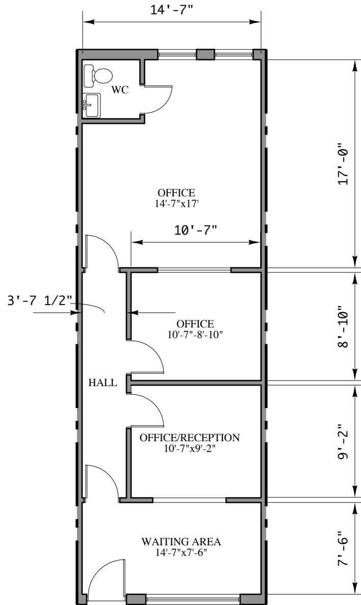
1 SUITE 215 SCALE: 1/8" = 1'-0"
