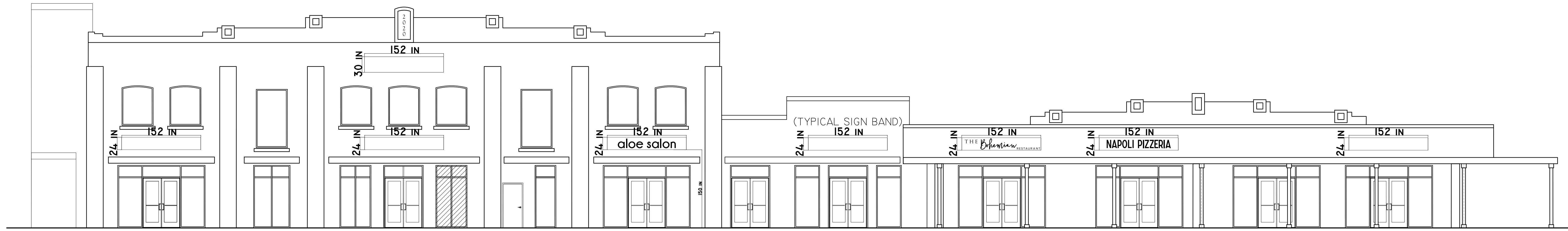
WEST (PRIMARY) ELEVATION SCALE: 1/8" = 1'-0"
