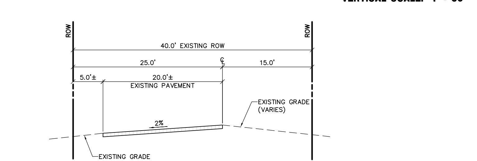
EL SUENO WAY A-1 SECTION HORIZONTAL SCALE: 1" = 10' VERTICAL SCALE: 1" = 2'
