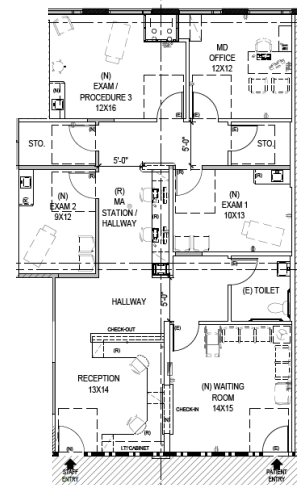
Suite 650 Test Fit Example:
