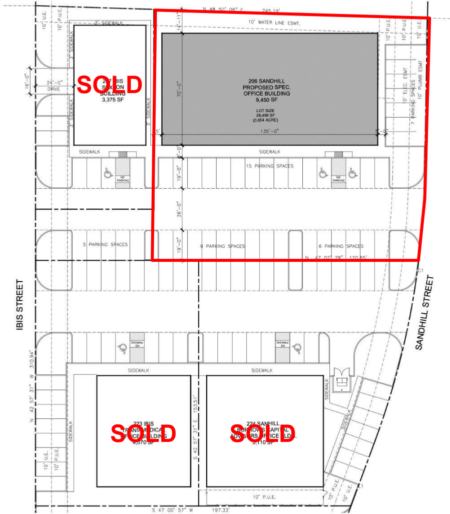
01 SITE PLAN SCALE 1/16"=1'-0"
