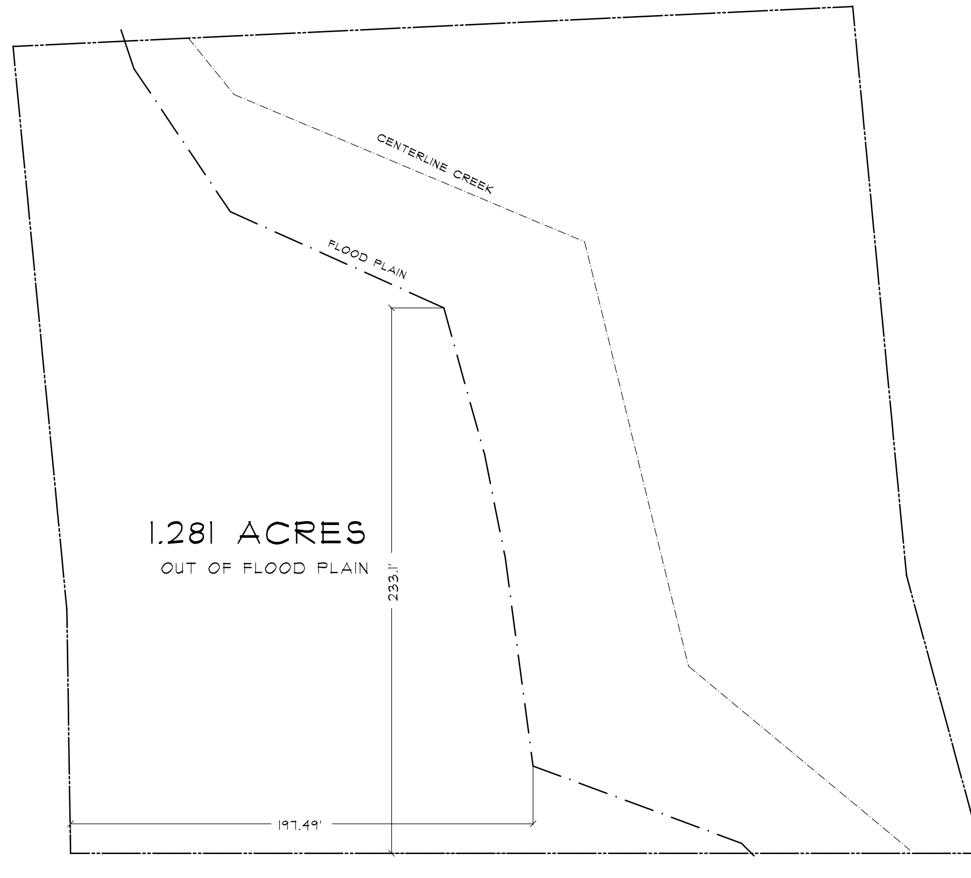
4401 TRIMMIER ROAD SITE PLAN 1:40
