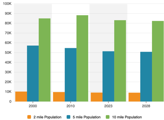
Population
