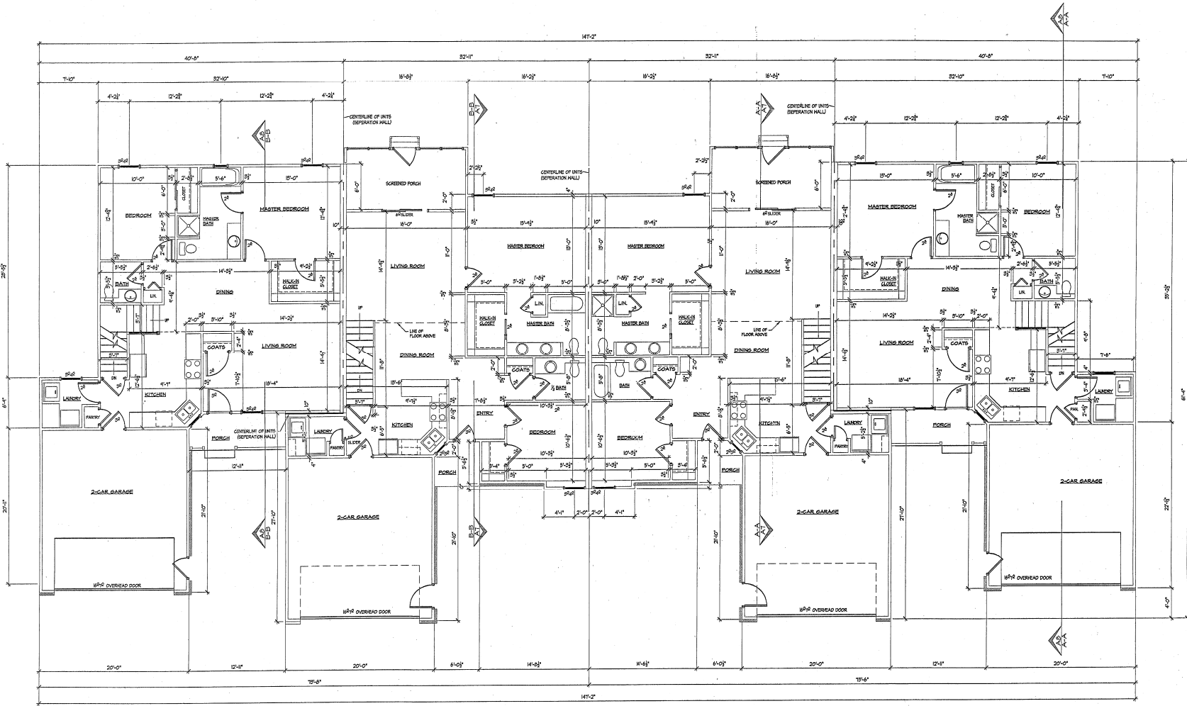
4-UNIT FLOOR PLAN B-A-A-B 178 SQFT/UNIT SCALE: 3/8" = 1'-0"
