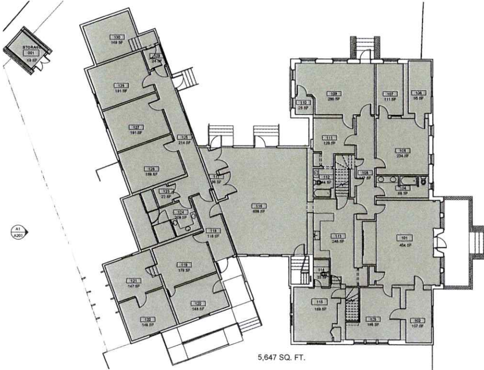
A1 A101 FIRST FLOOR SCALE: 1/8" = 1'-0"
