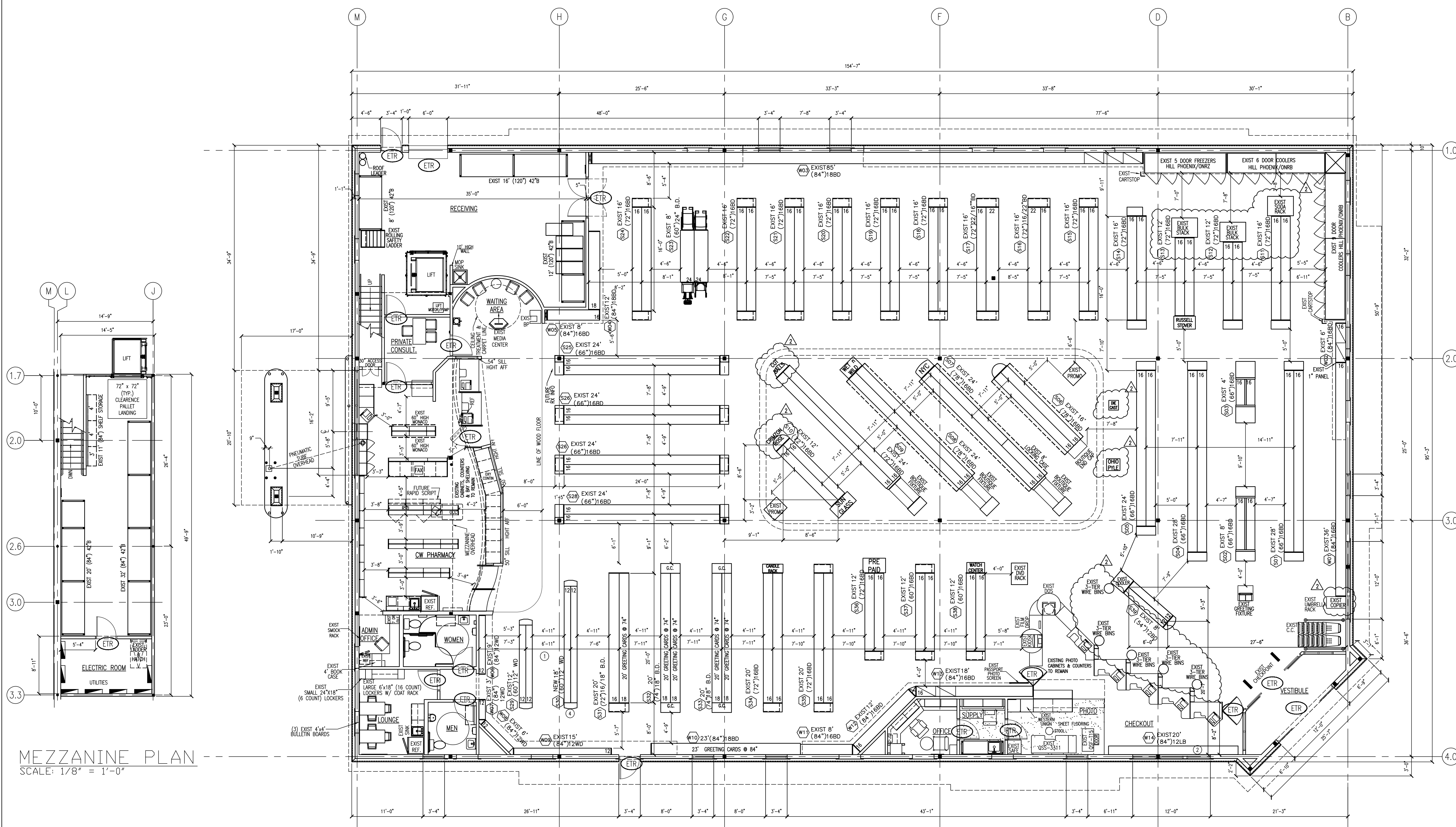
FIXTURE PLAN SCALE: 1/8" = 1'-0"
