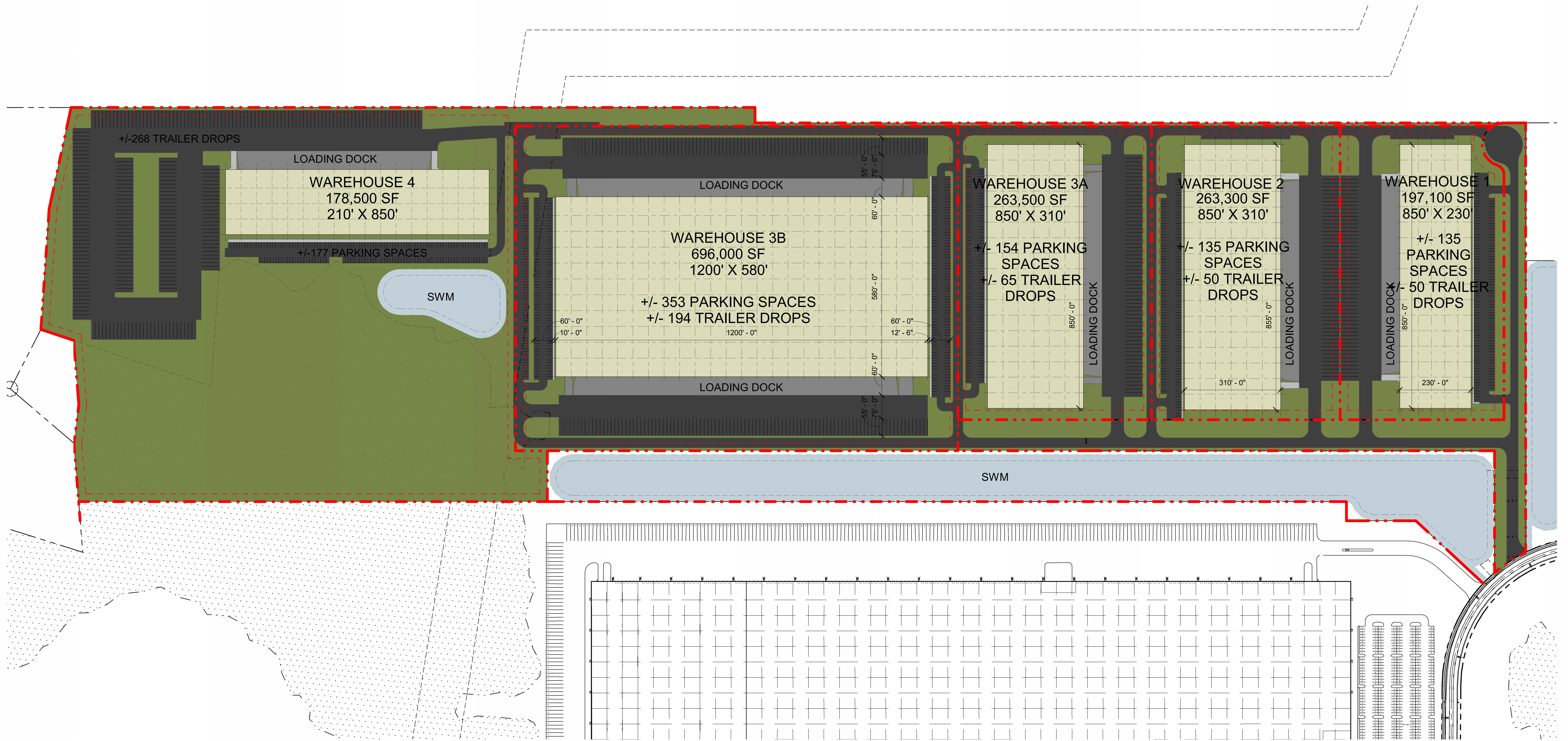
1 SITE PLAN - OPTION 13A 1 : 1600
