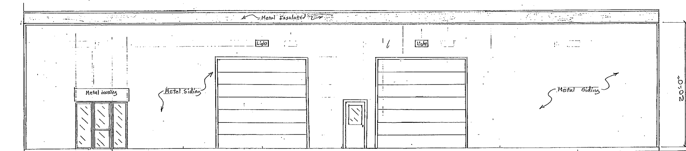
Right-Side Scale: 1/4"=1'-0"
