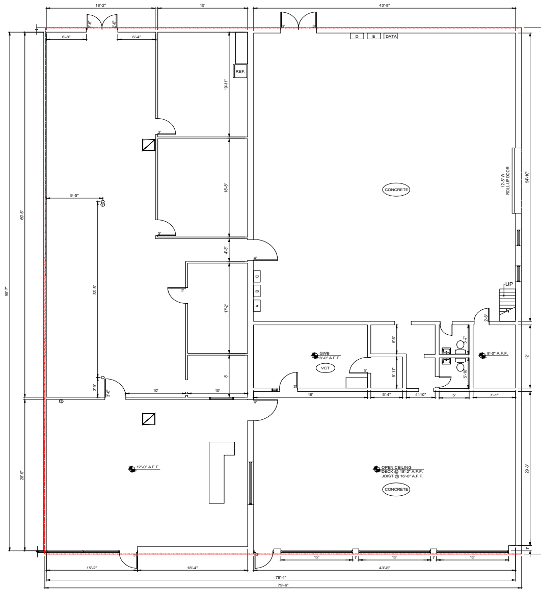
FIRST FLOOR PLAN N.T.S.
