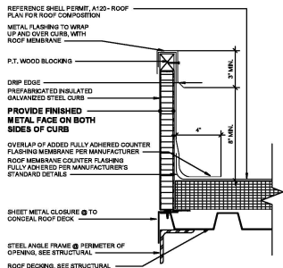
4 ROOF MECHANICAL CURB SCALE: 3" = 1'-0" | ARCO: A01.04
