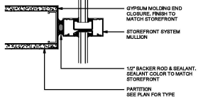
3 PARTITION AT MULLION SCALE: 3" = 1'-0" | ARCO: 131.01
