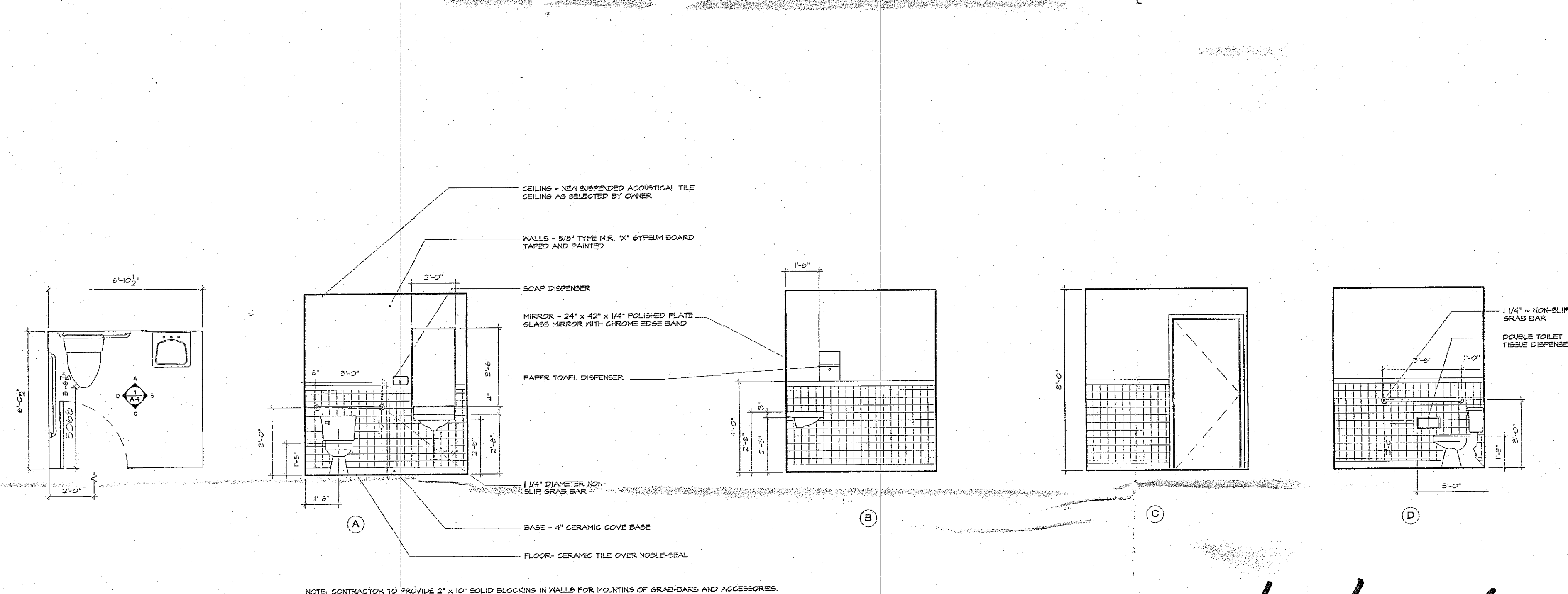
2 H.C. BATHROOM A-1 N.T.S. ♦
