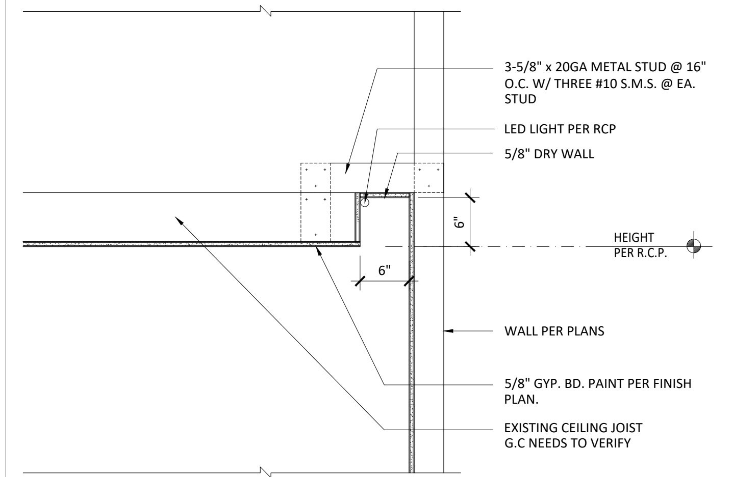
2 COVE DETAIL SCALE: 1" = 1'-0"
