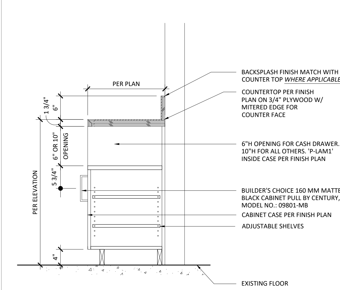
2 CABINET W/ BACKSPLASH SCALE: 1" = 1'-0"
