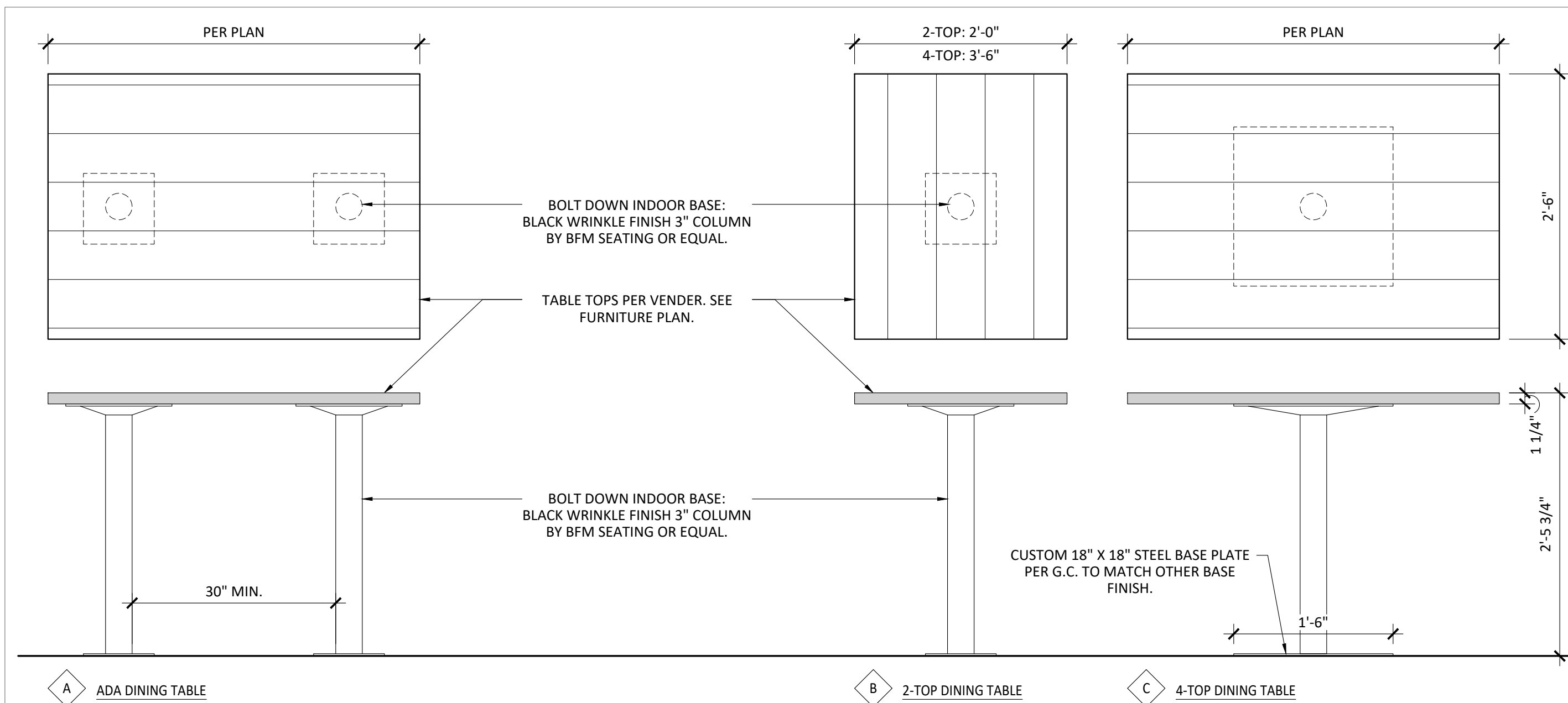
4 DINING TABLE DETAILS SCALE: 1" = 1'-0"
