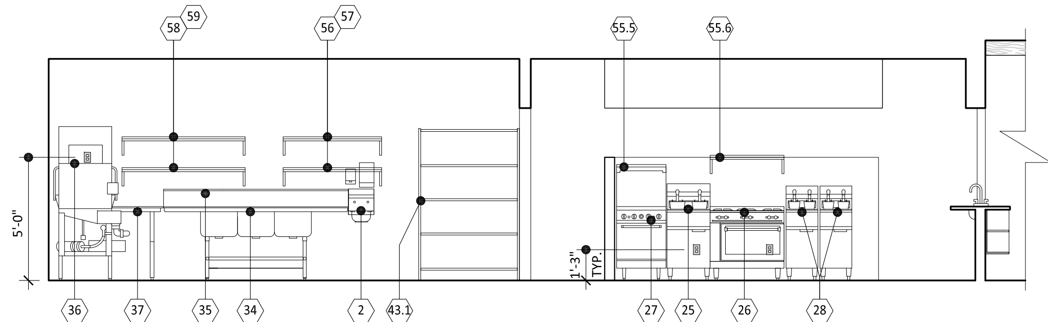
4 ELEVATION
