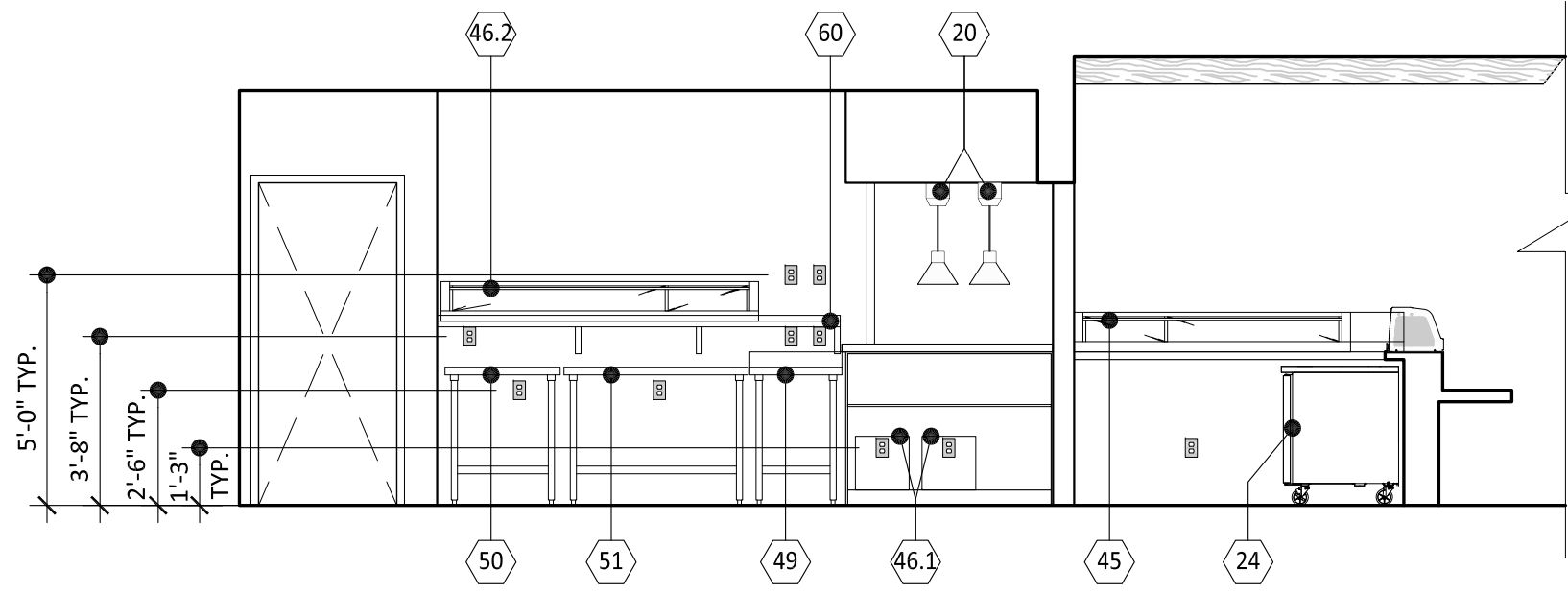
2 ELEVATION
