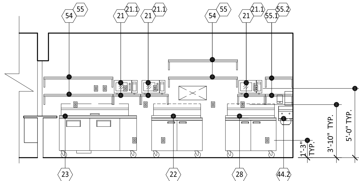
5 ELEVATION
