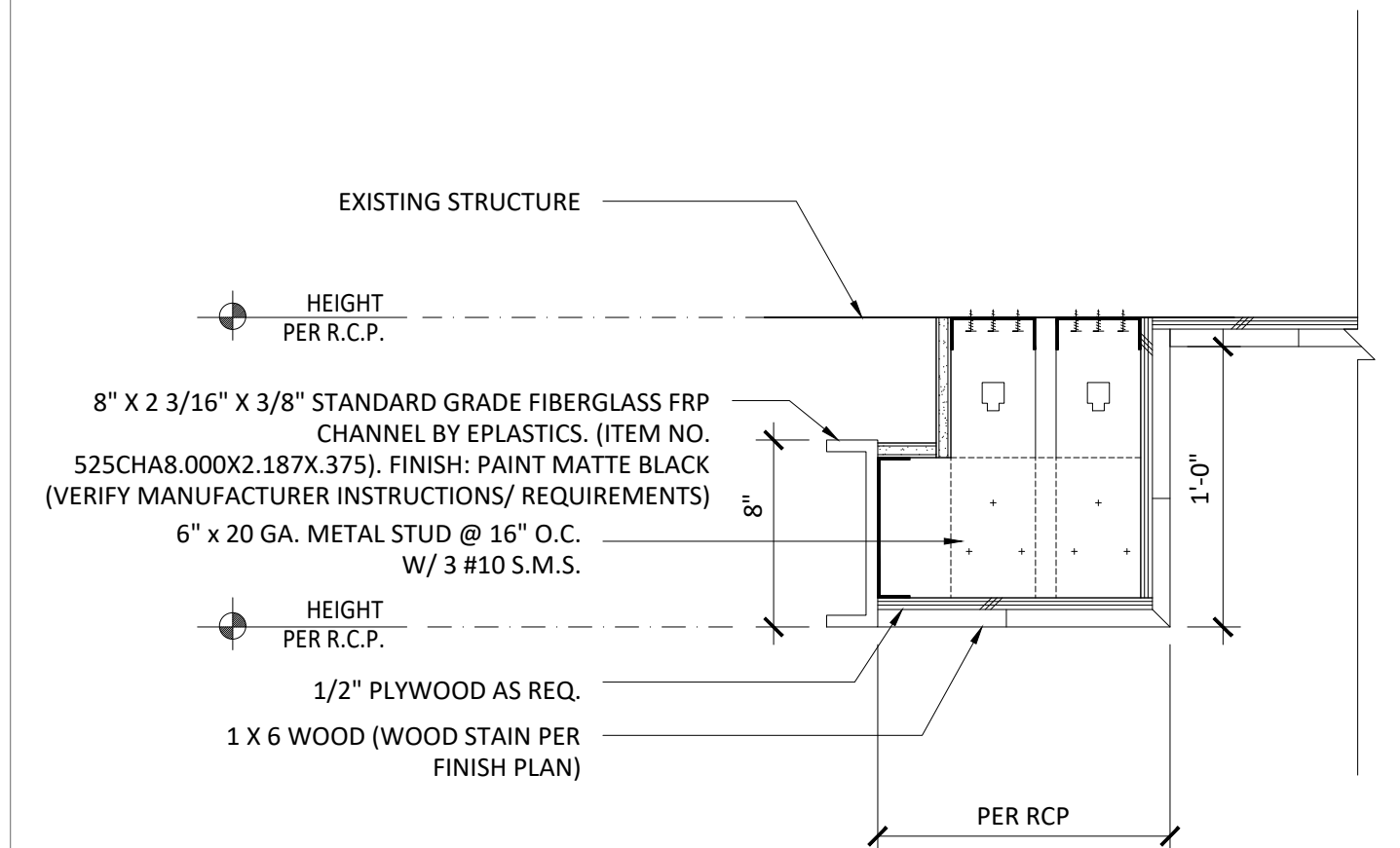
3 SOFFIT DETAIL @ BAR SCALE: 1-1/2" = 1'-0"
