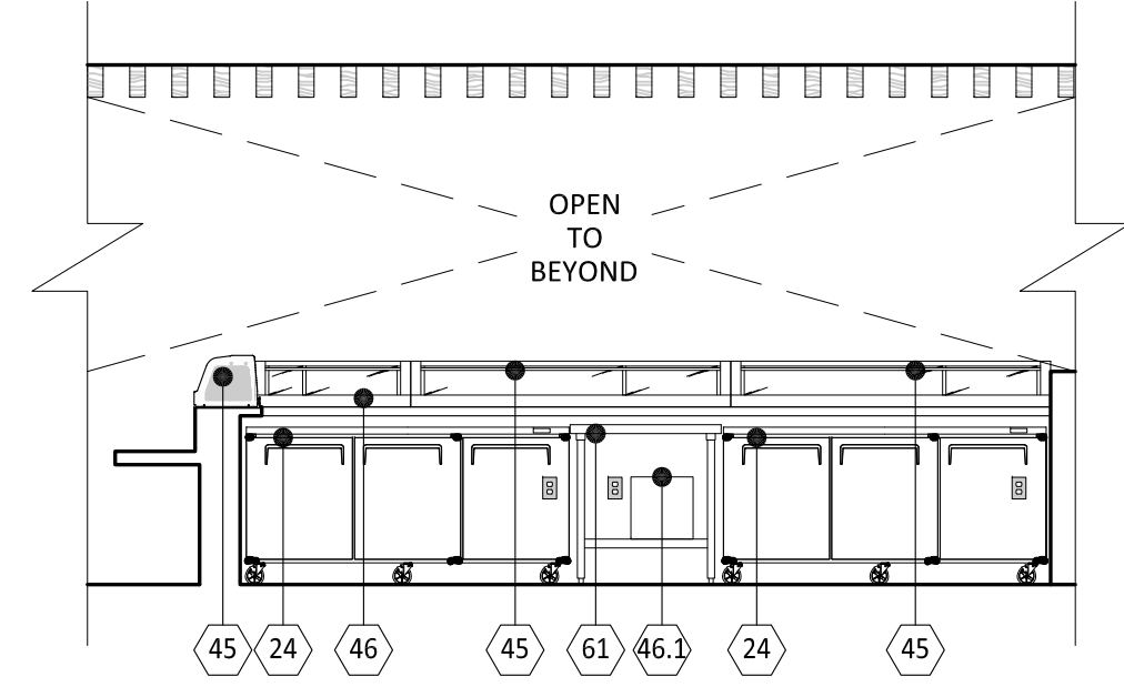
1 ELEVATION
