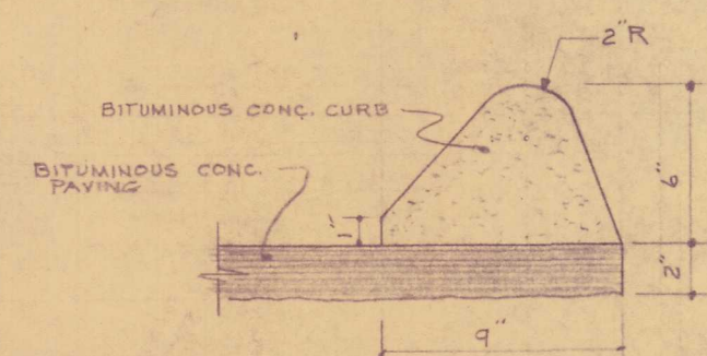
BITUMINOUS CONC. CURB SCALE: 1/2" = 1'-0"
