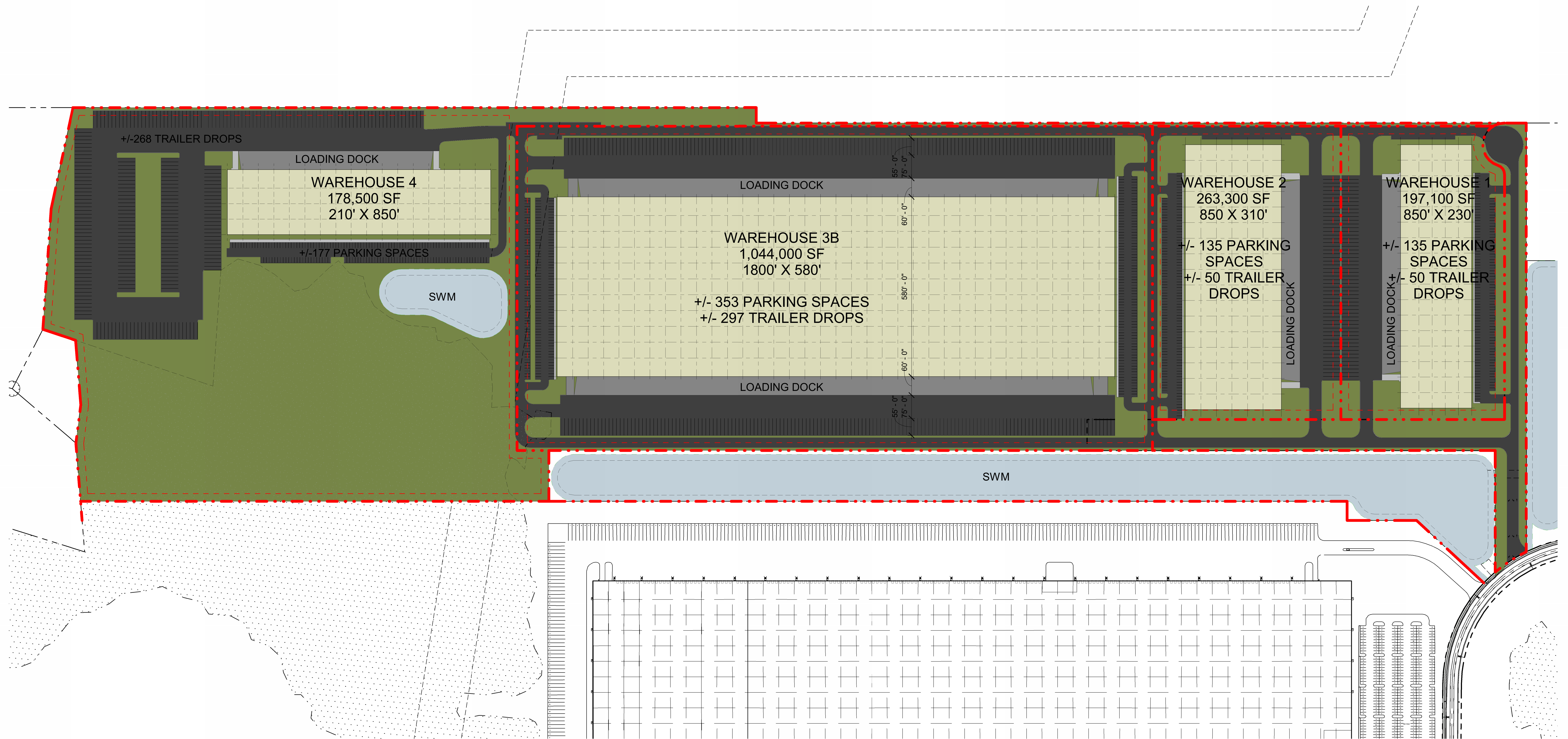
1 SITE PLAN - OPTION 13B 1 : 1600
