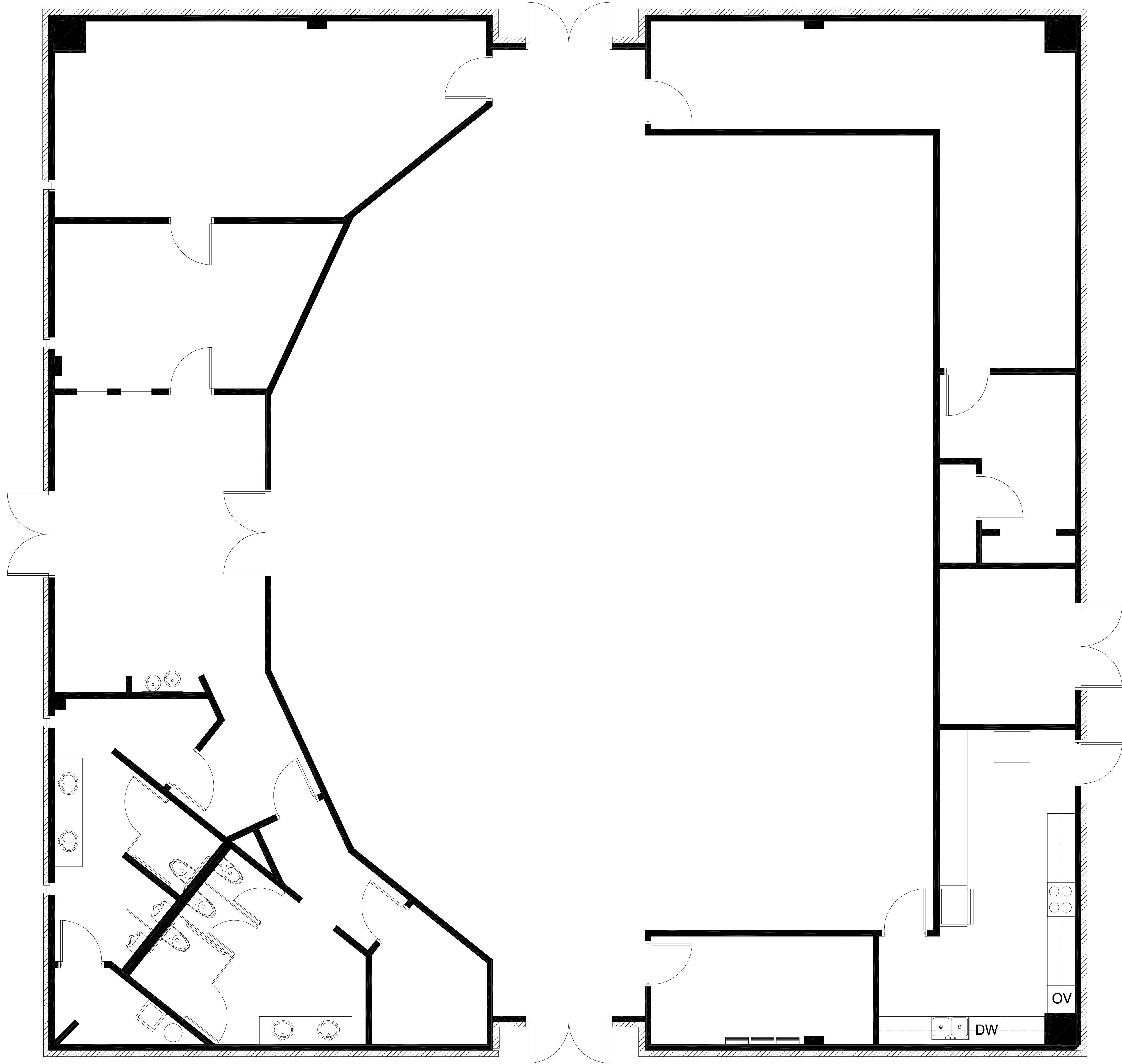
01 FLOORPLAN SCALE: 1/4" = 1'-0"
