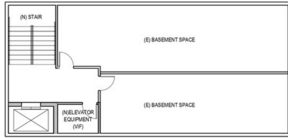
SUITE 180 BASEMENT SPACE PLAN
