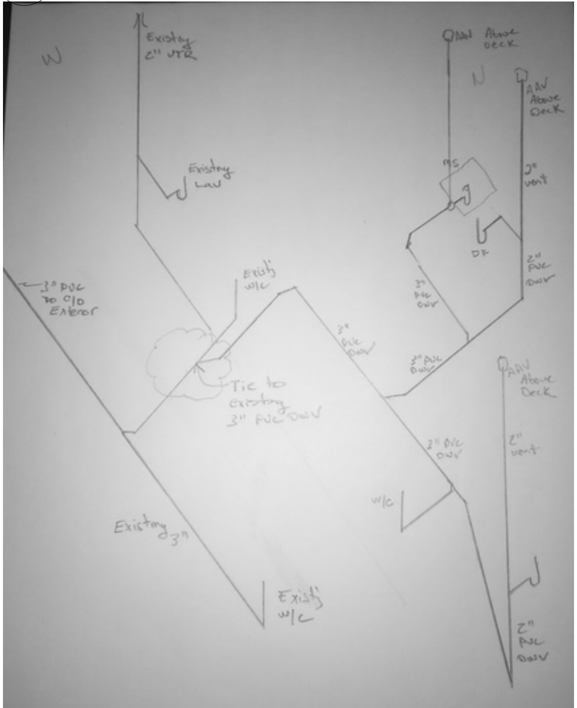
4 A-2 PLUMBING RISER DIAGRAM SCALE: 1/4" = 1'-0"
