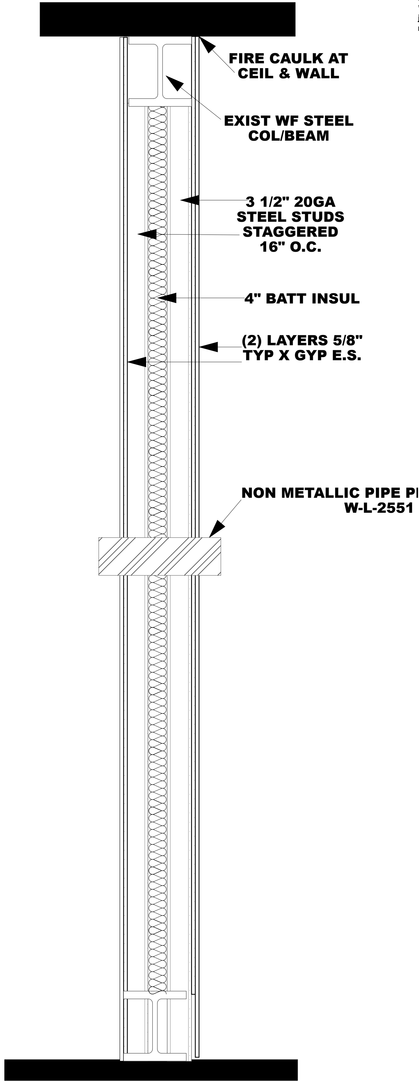
5 A-2 2 HR WALL SECTION SCALE: 1" = 1'-0"
